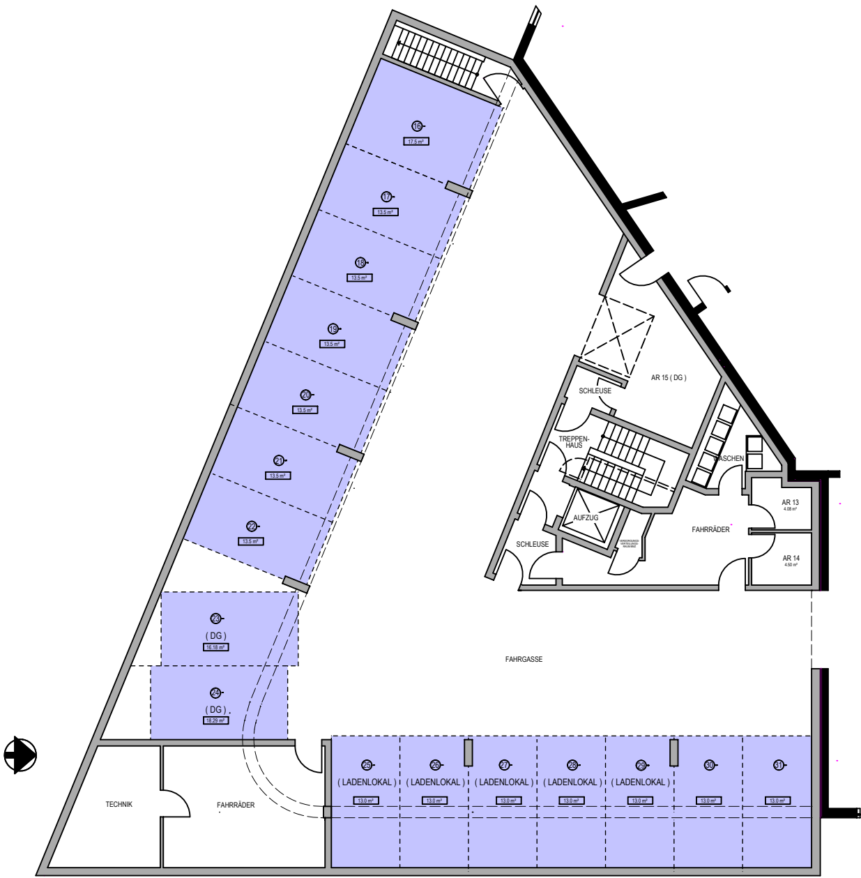
KELLERGESCHOSS / TIEFGARAGE
